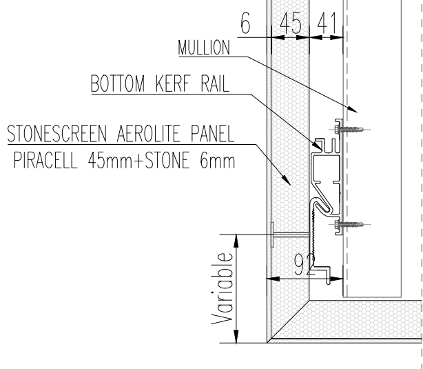
S4 Kerf Rails NTS @A4
